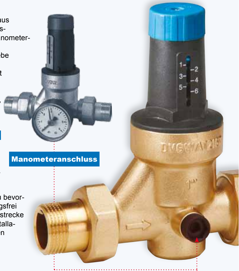
Drehknopf
