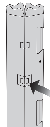
2.) Darunterliegende, zweifach gelochte Stabhalterung, kreisbogenförmig herausziehen und mittig knicken, sodass die Löcher deckungsgleich übereinander liegen.
